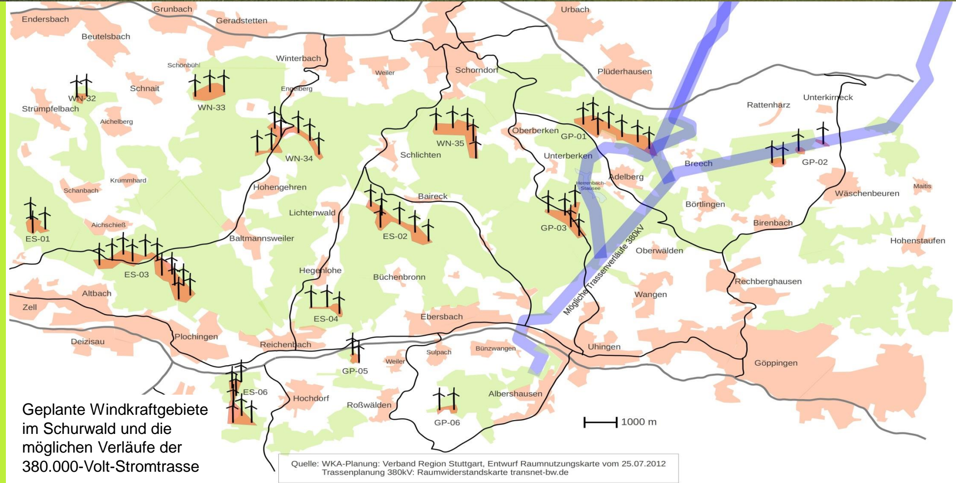
Wäschenbeuren geplanter Windpark und die geplante 380.000-Volt-Stromtrasse
