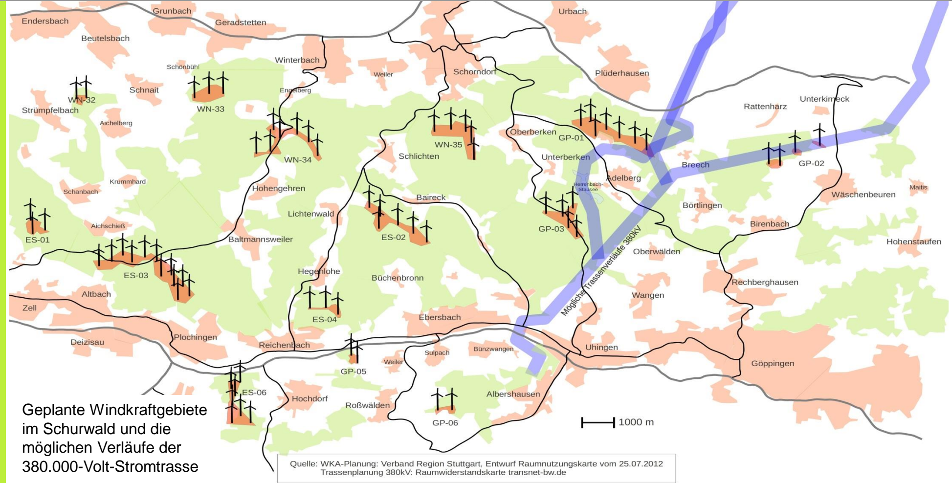
Windkraftanlagen um Adelberg und die geplante 380.000-Volt-Stromtrasse
