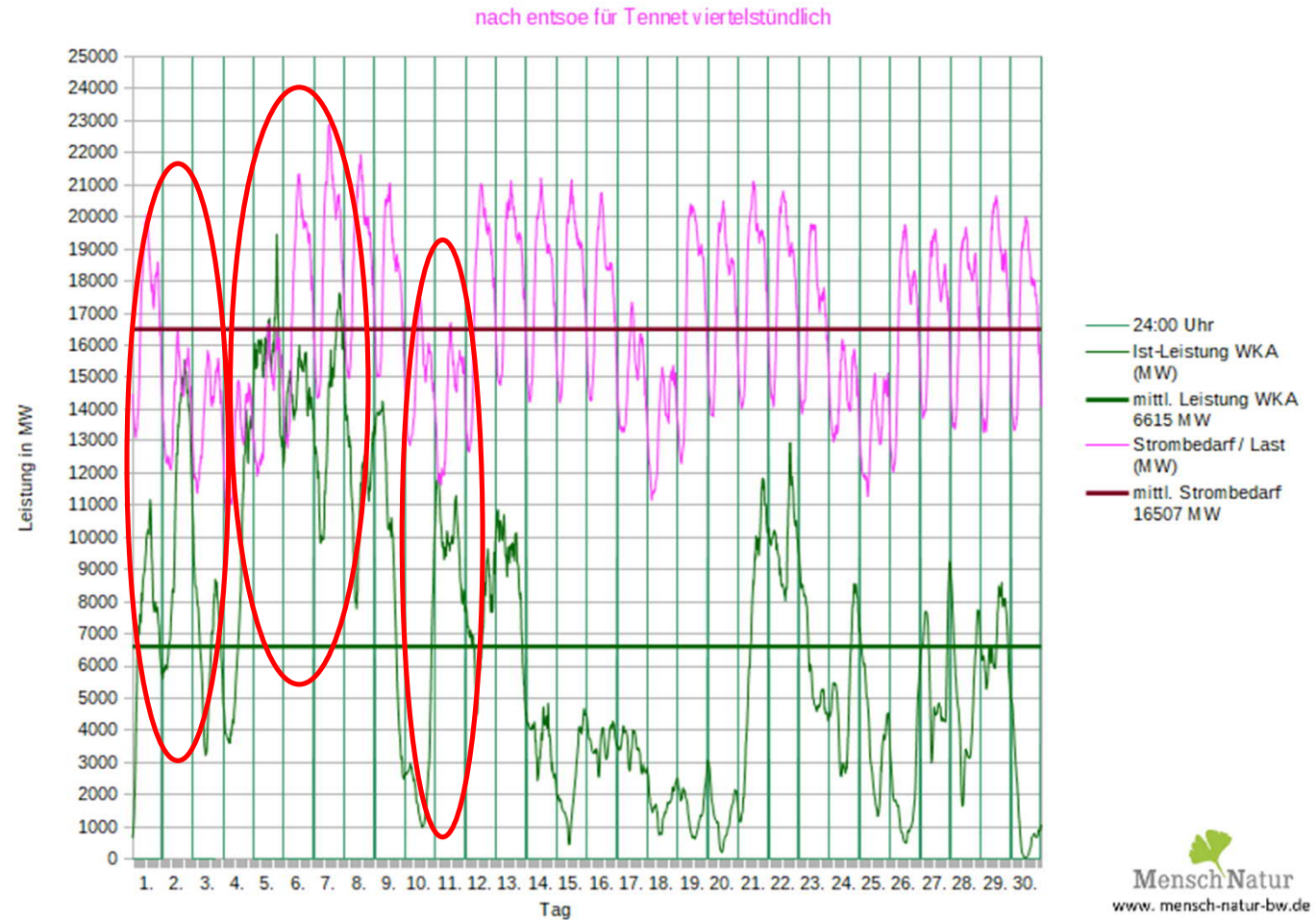
Leistungsverlauf aller WKA im Netz von Tennet gegenüber Strombedarf / Lastanforderung im April 2021
