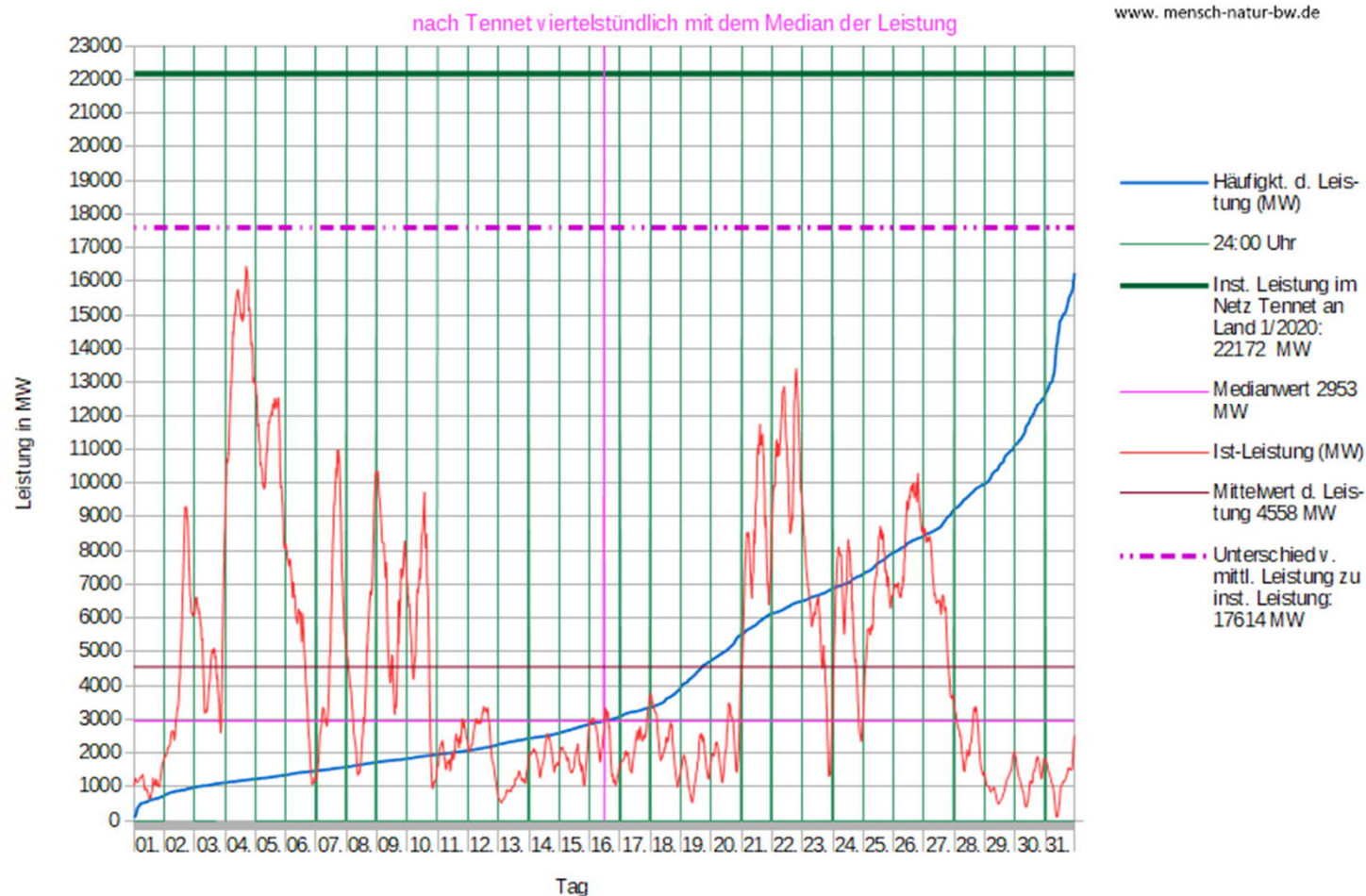
Leistungsverlauf aller WKA an Land im Netz Tennet im Mai 2021
