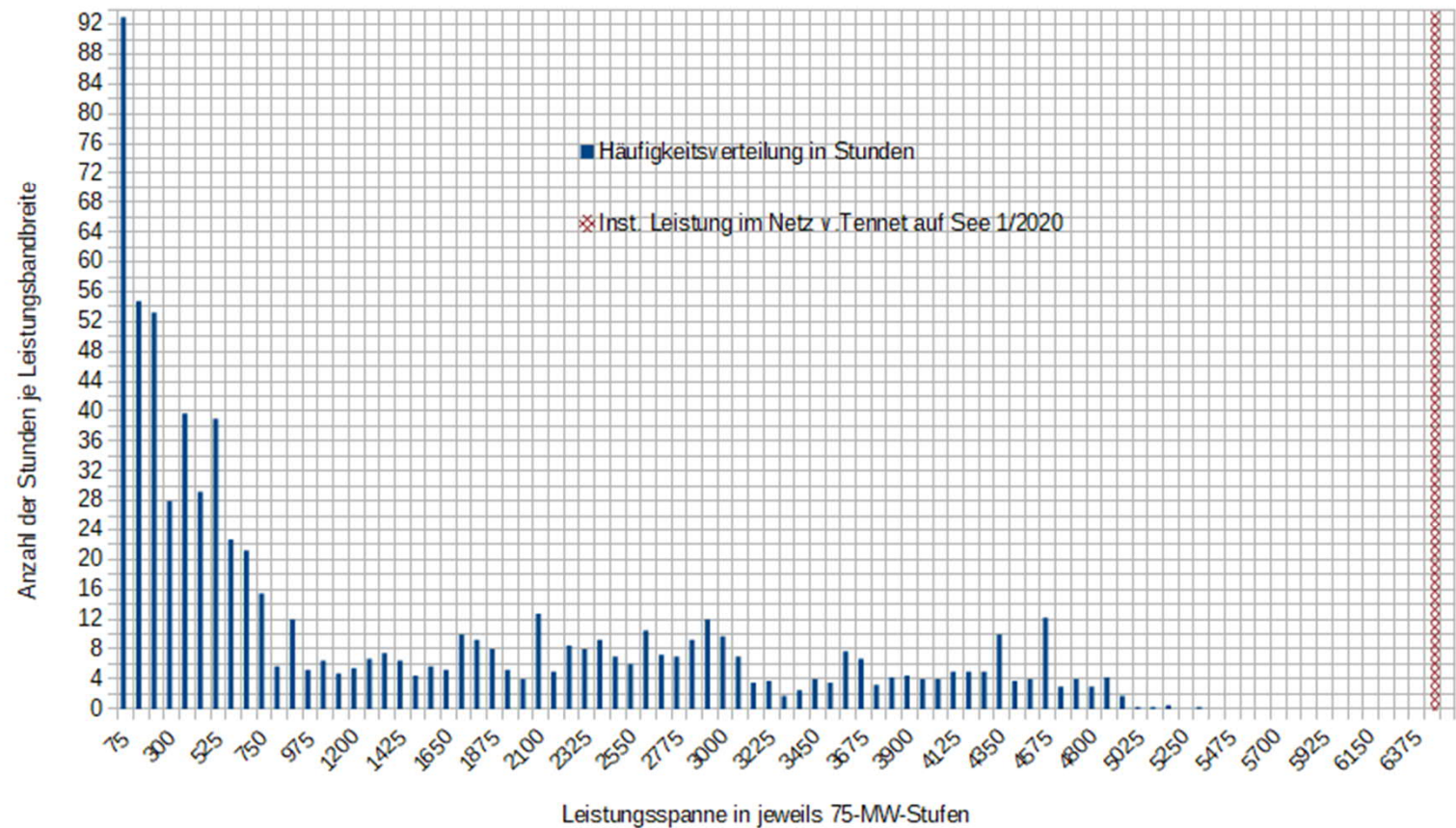
Häufigkeitsverteilung der Leistung auf See Tennet
