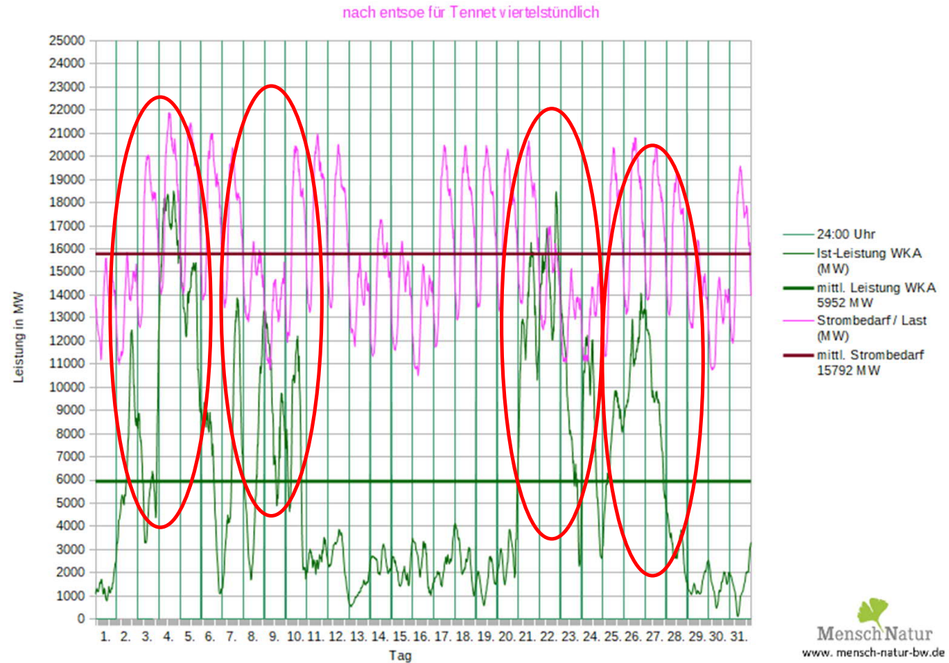
Leistungsverlauf aller WKA im Netz von Tennet gegenüber Strombedarf / Lastanforderung im Mai 2021
