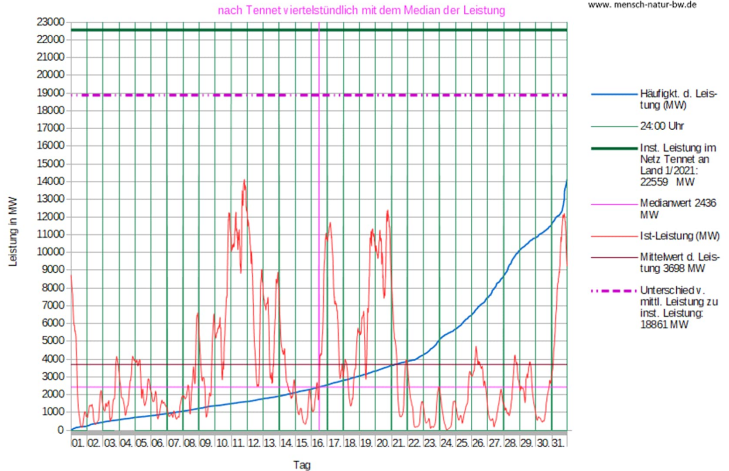
Leistungsverlauf aller WKA an Land im Netz Tennet im März 2022
