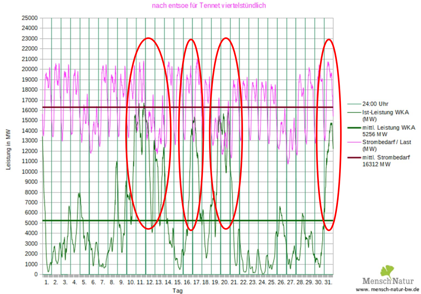
Leistungsverlauf aller WKA im Netz von Tennet gegenüber Strombedarf / Lastanforderung im März 2022
