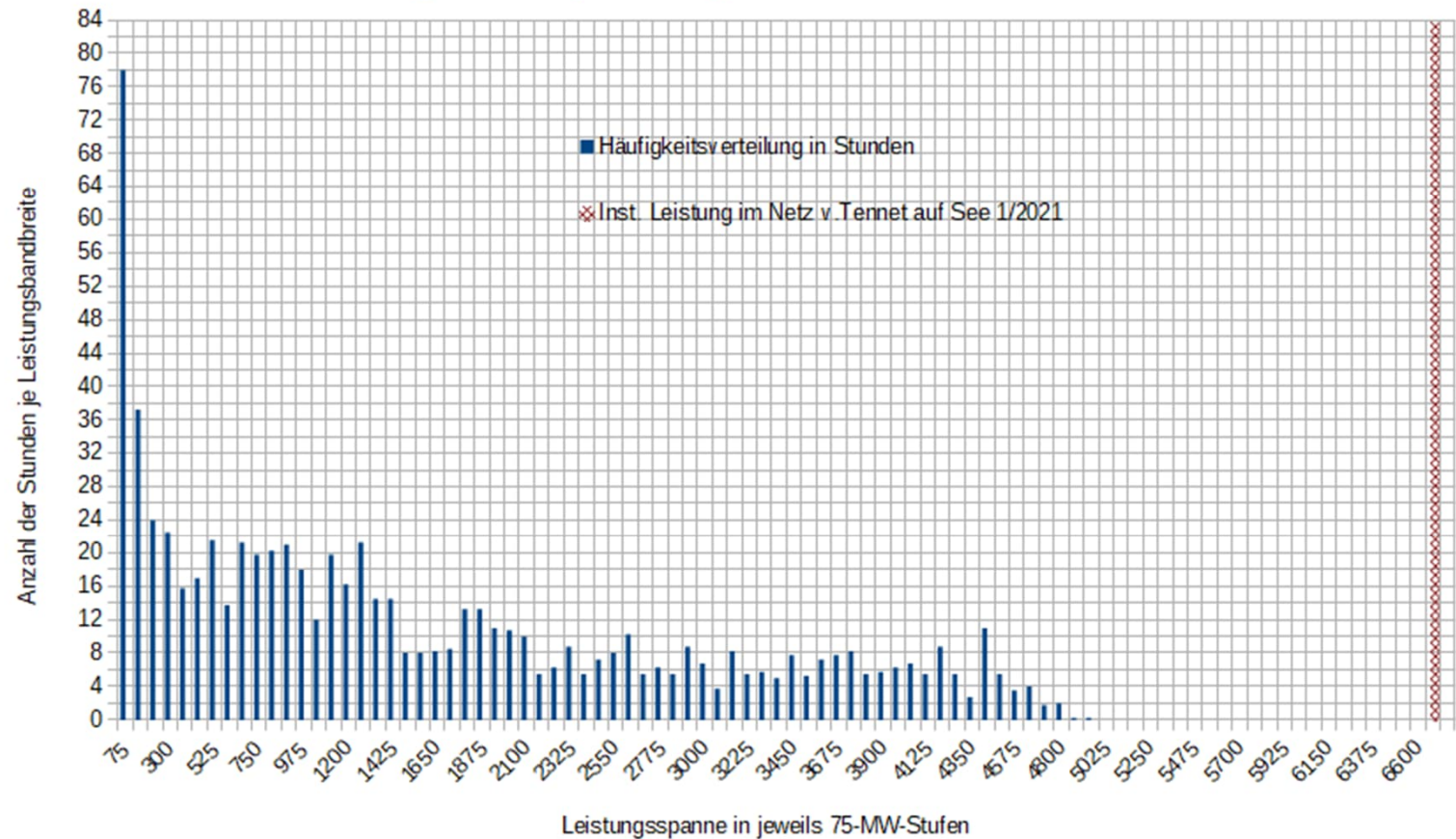
Häufigkeitsverteilung auf See über die monatliche Gesamtstunden mit verfügbaren Leistungsstufen in Stunden Tennet
