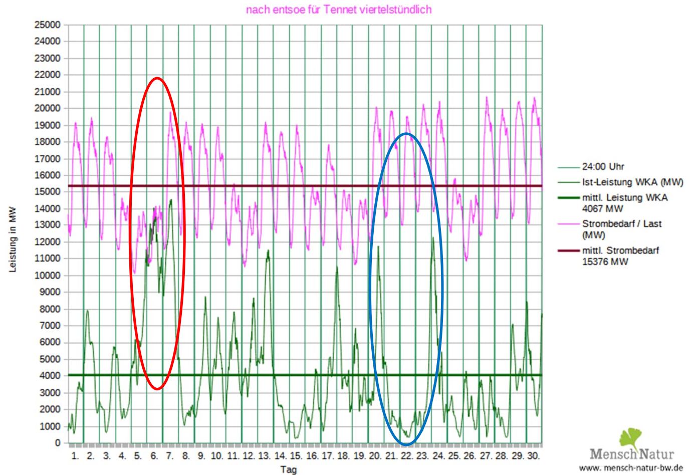
Leistungsverlauf aller WKA im Netz von Tennet gegenüber Strombedarf / Lastanforderung im Juni 2022
