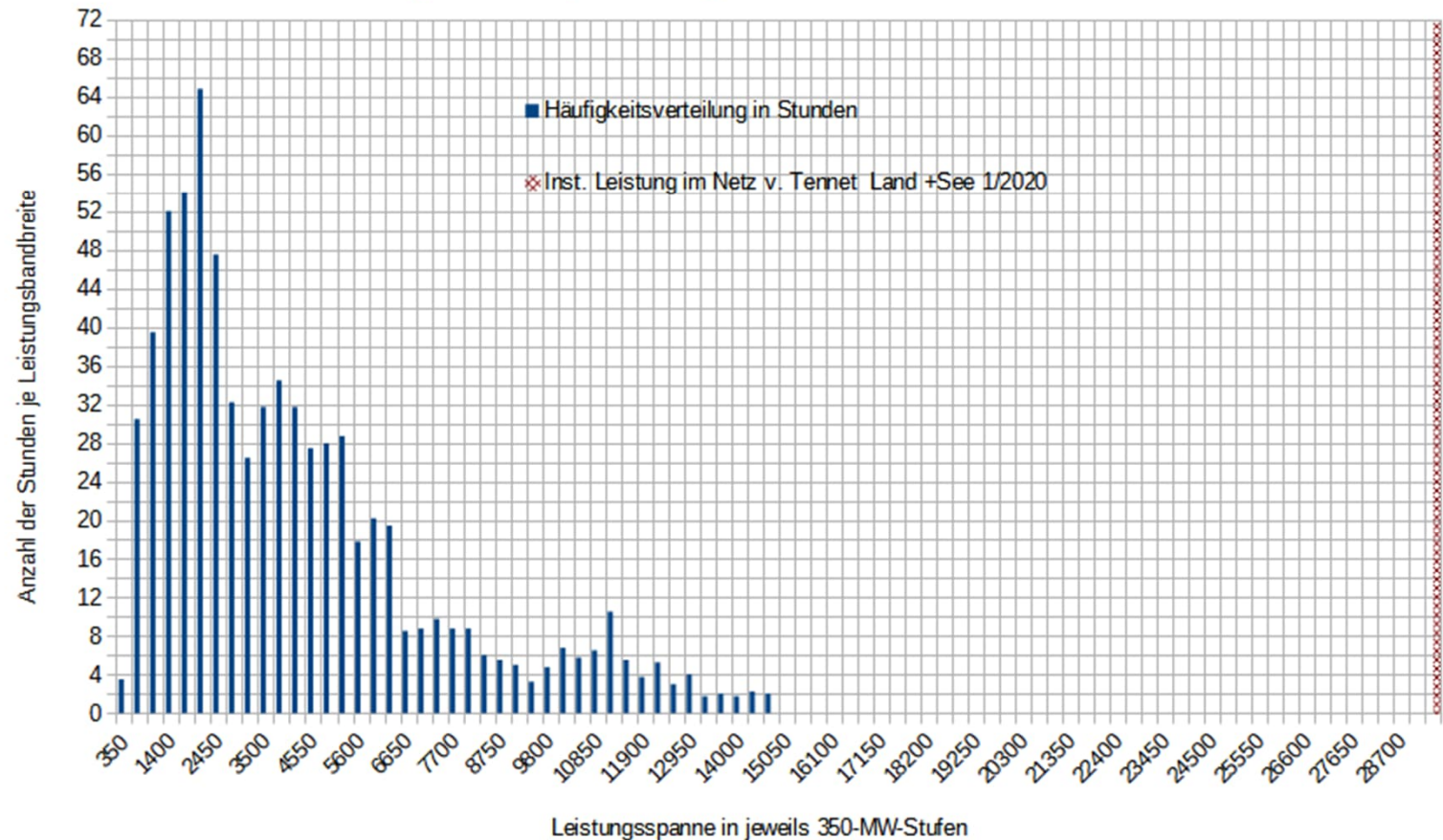
Häufigkeitsverteilung der Leistung Land und See Tennet
