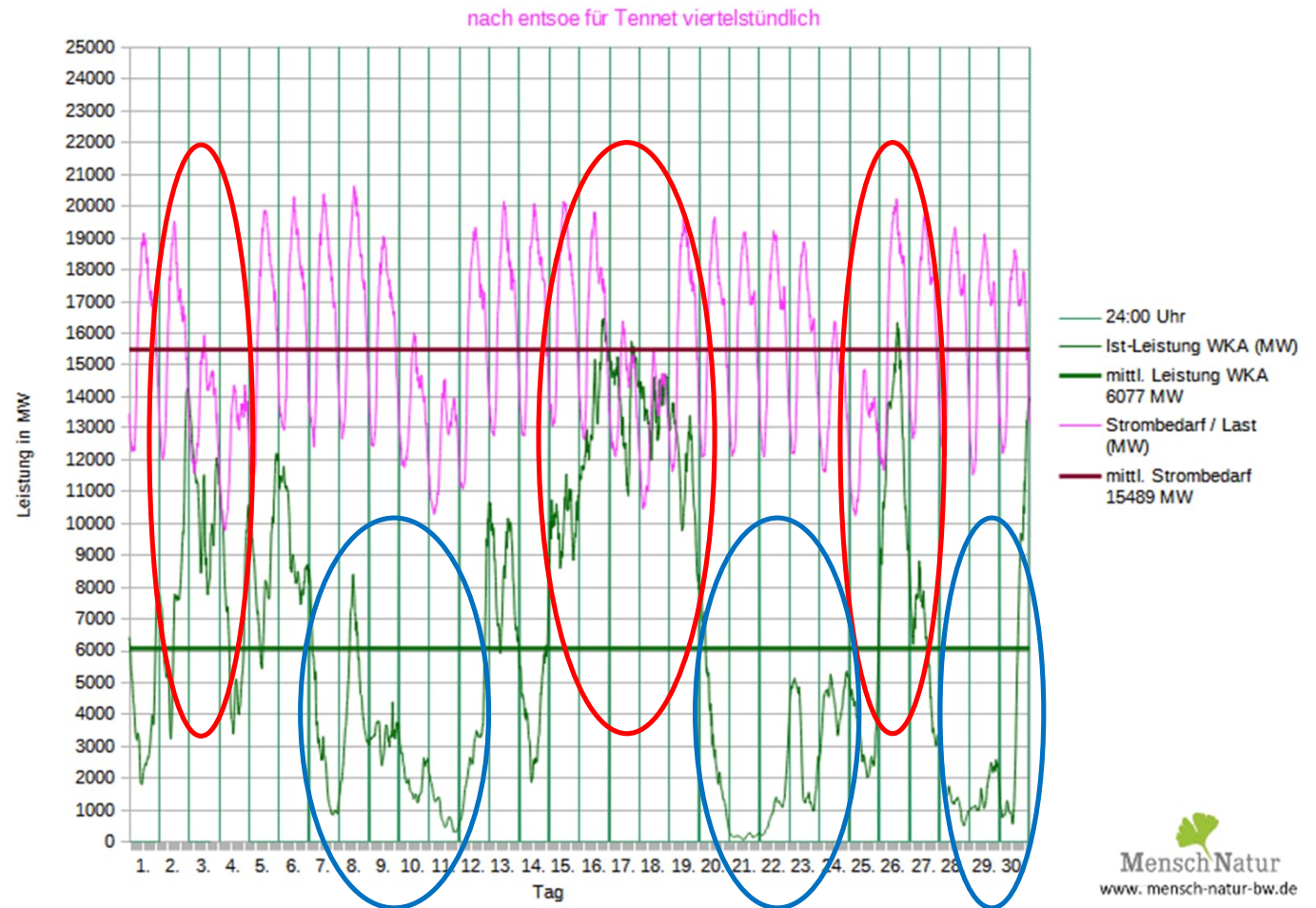
Leistungsverlauf aller WKA im Netz von Tennet gegenüber Strombedarf / Lastanforderung im September 2022
