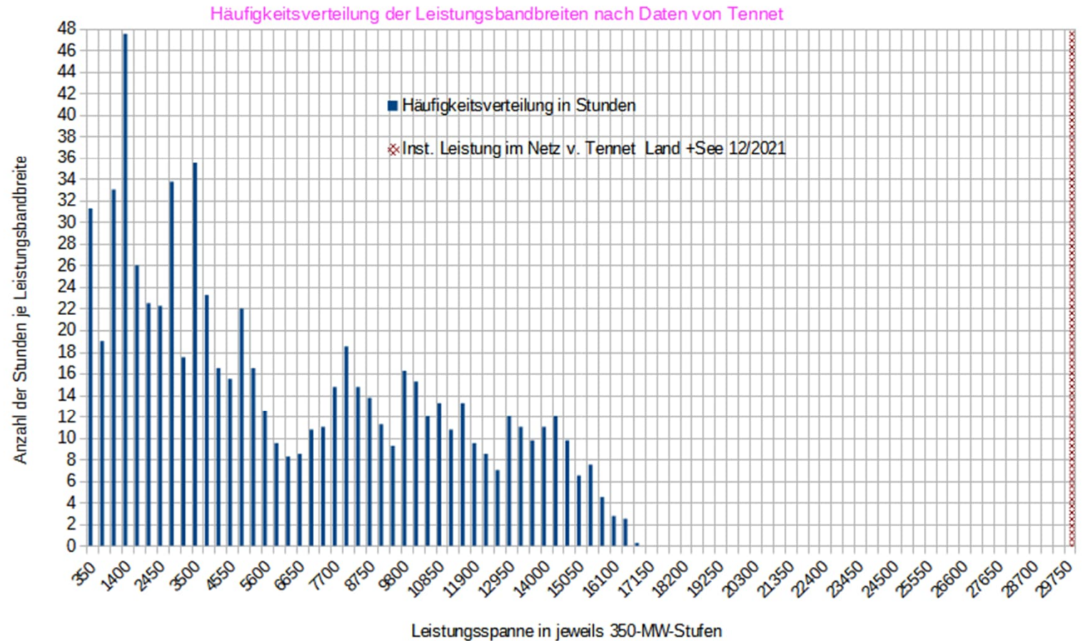
Häufigkeitsverteilung der Leistung Land und See Tennet
