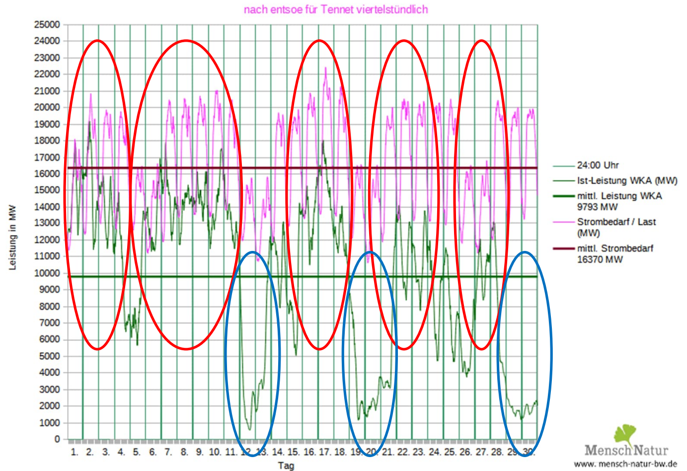
Leistungsverlauf aller WKA im Netz von Tennet gegenüber Strombedarf / Lastanforderung im November 2022
