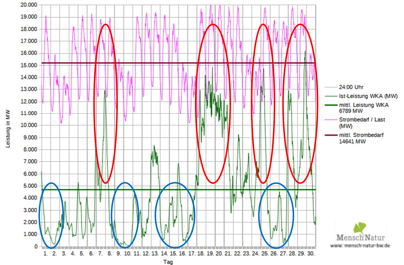
Leistungsverlauf aller WKA im Netz von Tennet gegenüber Strombedarf / Lastanforderung im September 2023
