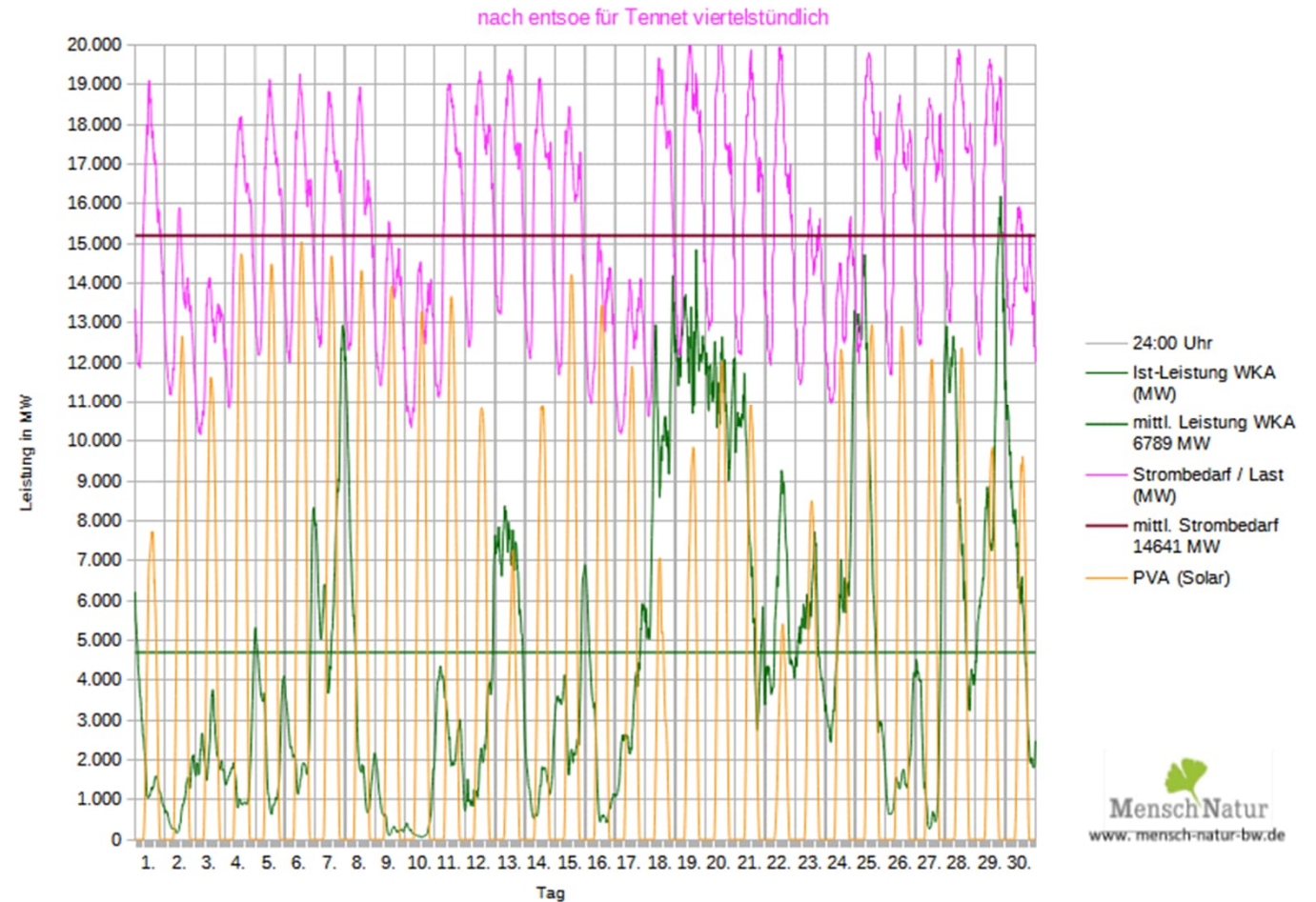
Leistungsverlauf aller WKA + PVA im Netz von Tennet gegenüber Strombedarf / Lastanforderung im September 2023
