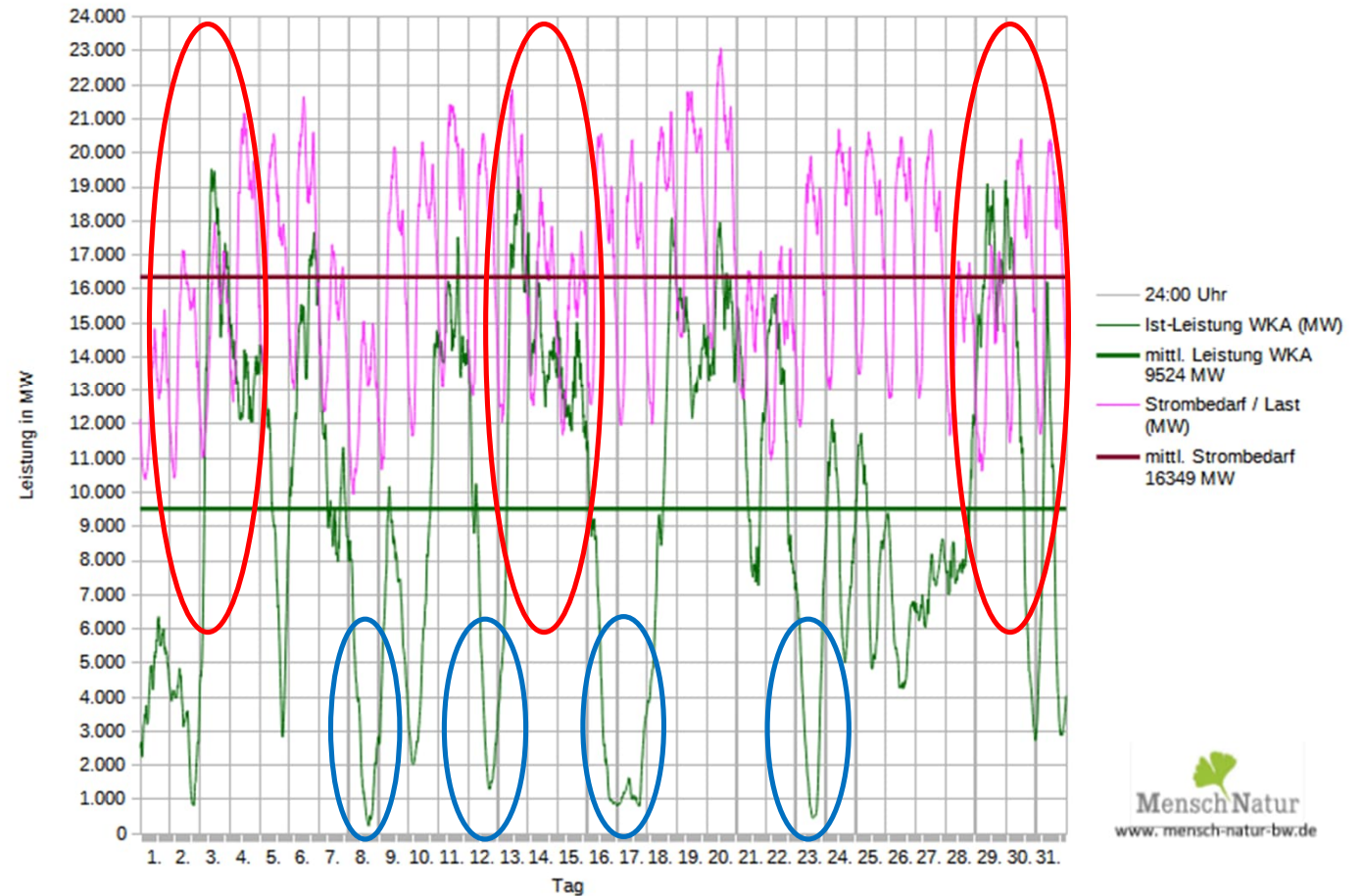
Leistungsverlauf aller WKA im Netz von Tennet gegenüber Strombedarf / Lastanforderung im Oktober 2023
