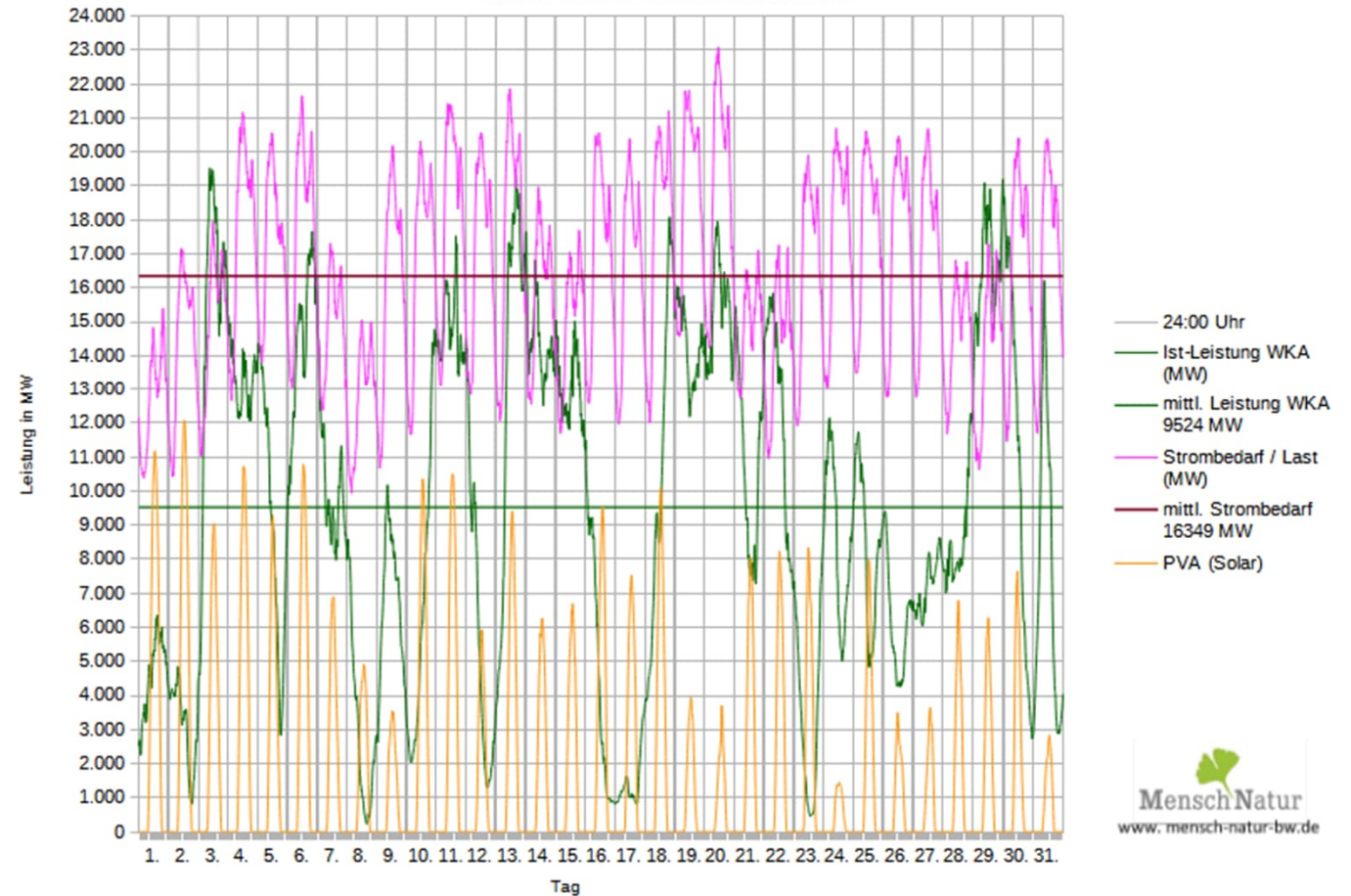
Leistungsverlauf aller WKA + PVA im Netz von Tennet gegenüber Strombedarf / Lastanforderung im Oktober 2023
