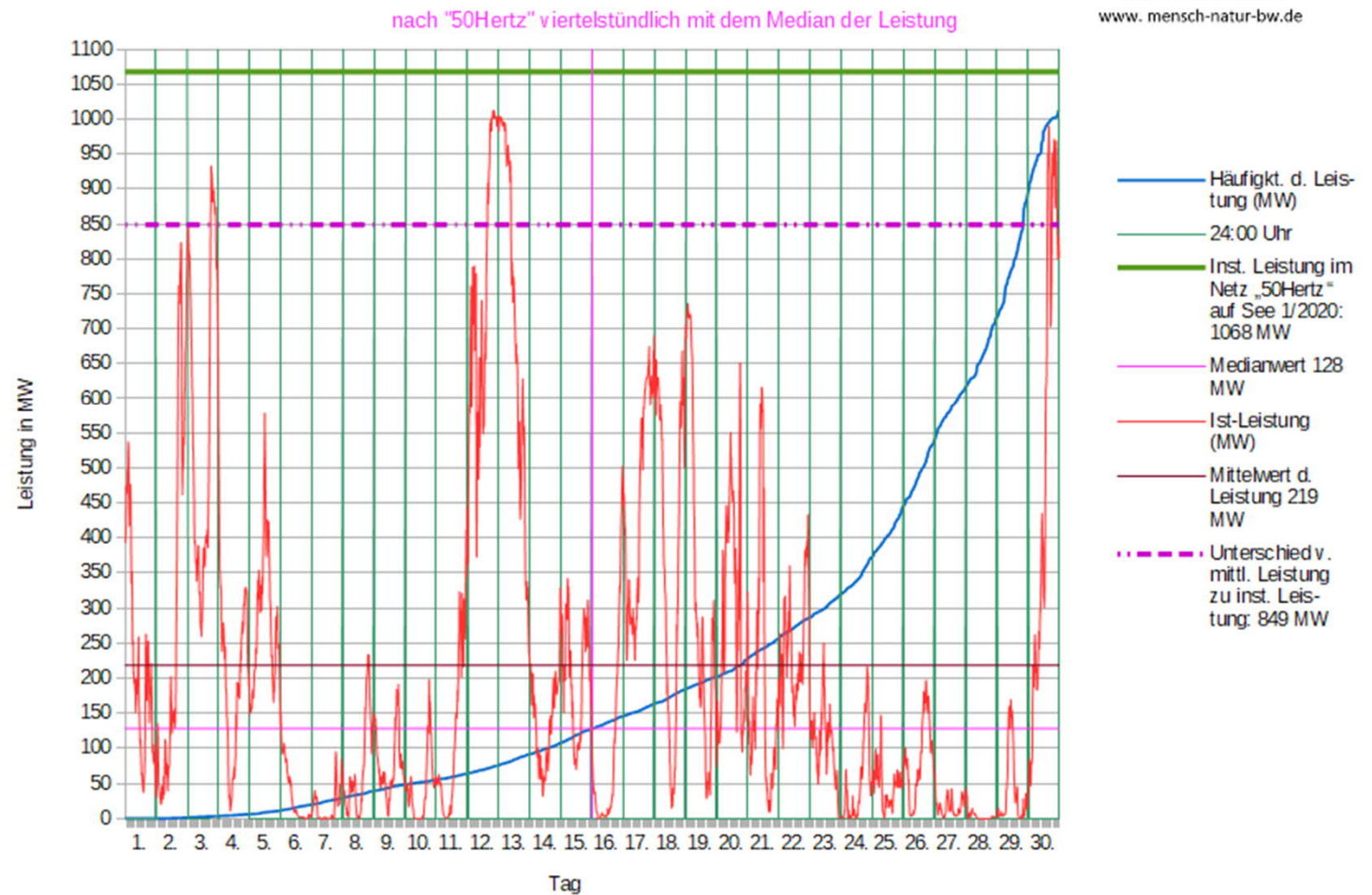
Leistungsverlauf aller WKA auf See im Netz "50Hertz" im Juni 2021
