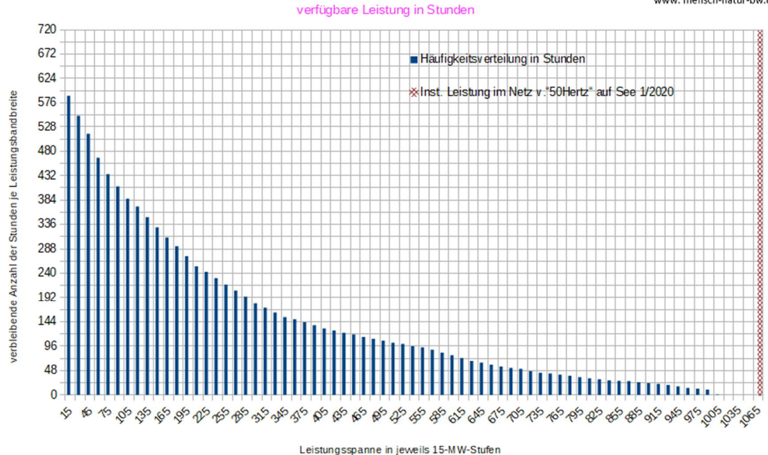
Häufigkeitsverteilung auf See über die monatliche Gesamtstunden mit verfügbaren Leistungsstufen in Stunden 50Hertz
