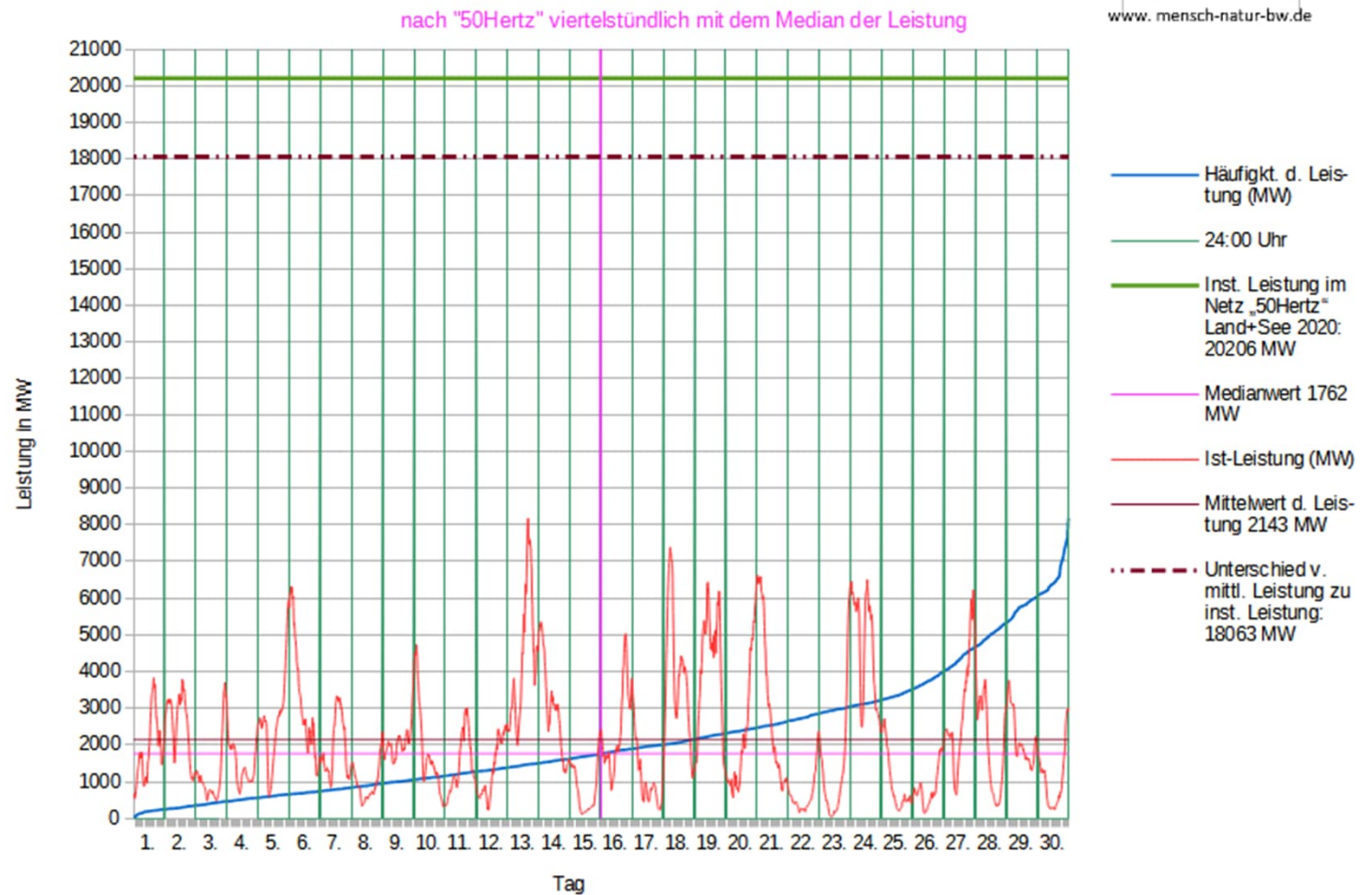
Leistungsverlauf aller WKA an Land + See im Netz "50Hertz" im Juni 2022
