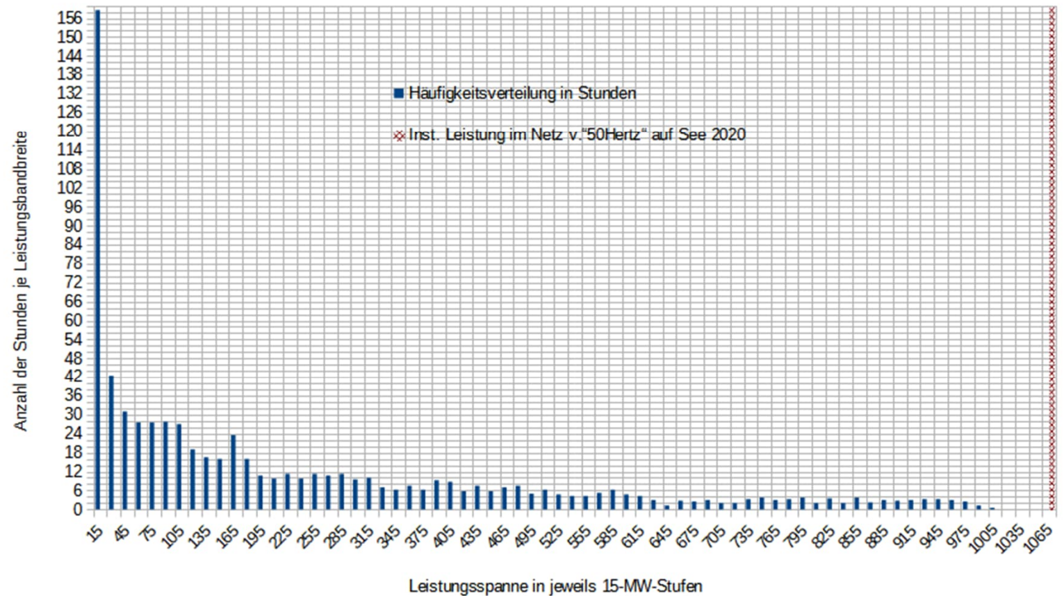
Häufigkeitsverteilung der Leistung auf See 50Hertz
