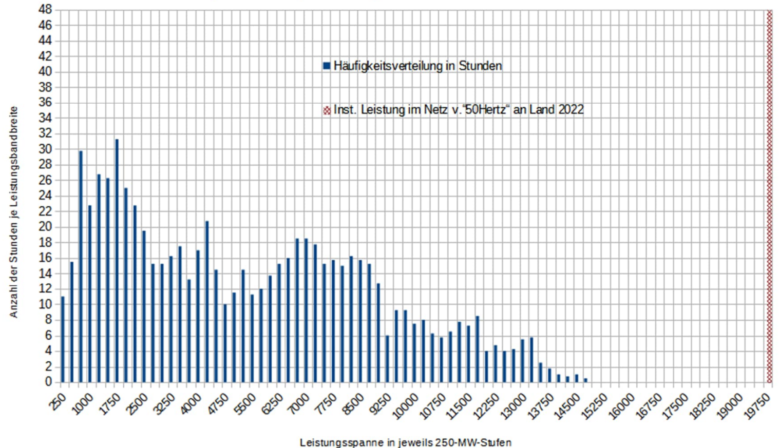
Häufigkeitsverteilung der Leistungsbreiten nach Daten von "50Hertz"
