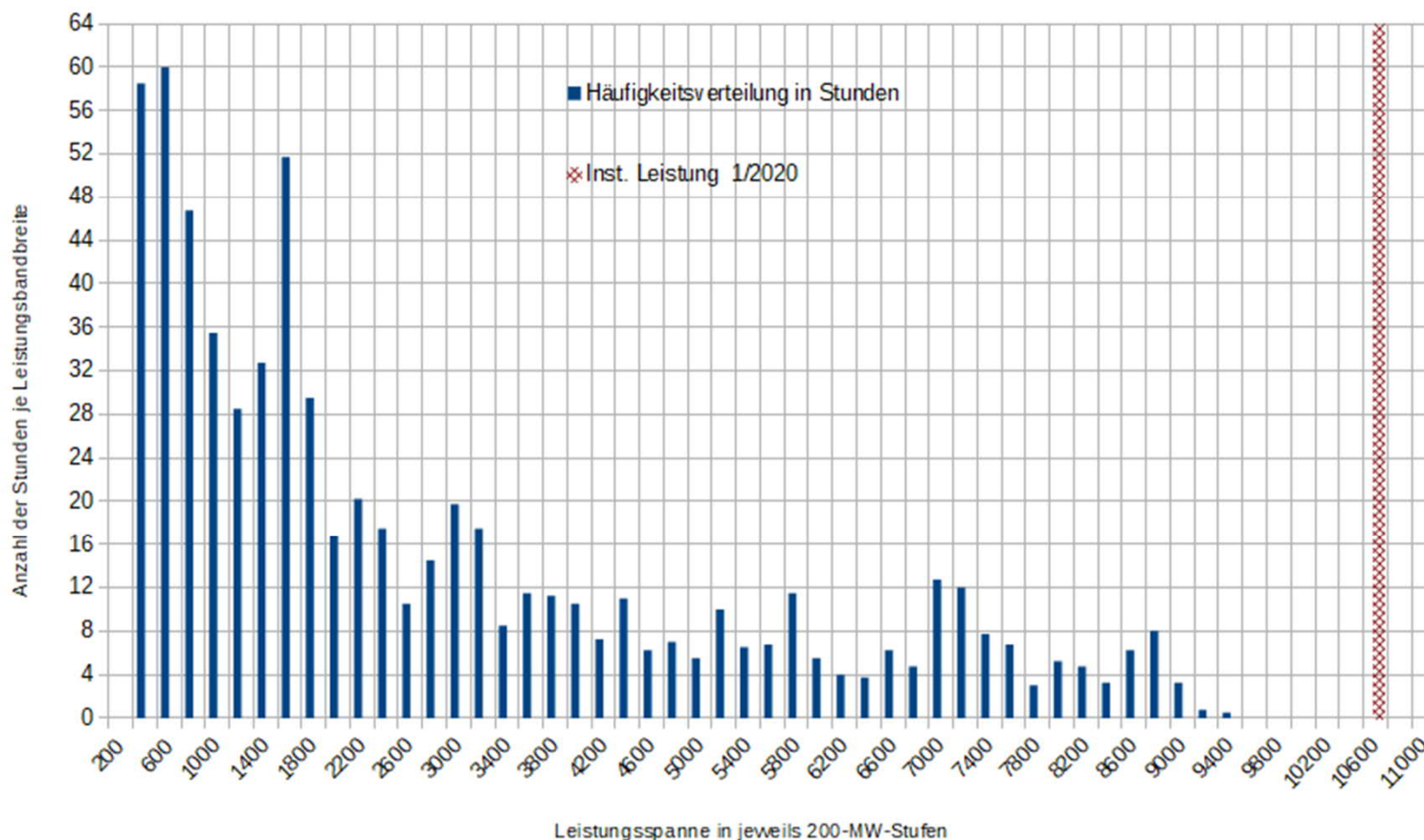
Häufigkeitsverteilung der Leistungsbandbreiten nach Daten von Amprion
