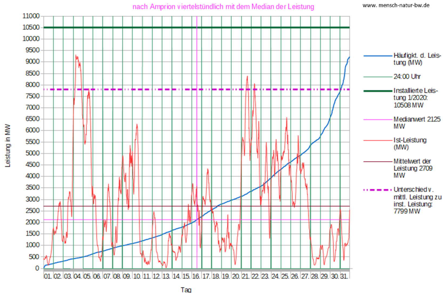
Analyse der Leistungsverteilung von Windenergie zur installierten Leistung Amprion
