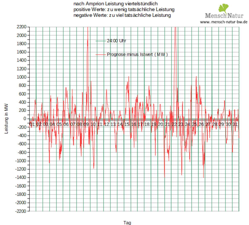
Differenz zw. Prognose der Leistung zu tatsächlicher Leistung in MW im Mai 2021
