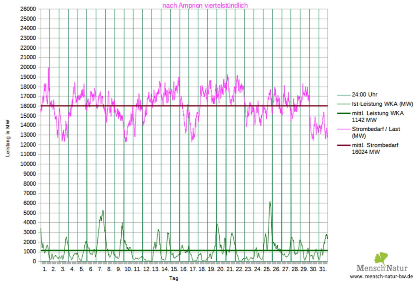
Leistungsverlauf Windleistung gegen Strombedarf (Last) Amprion
