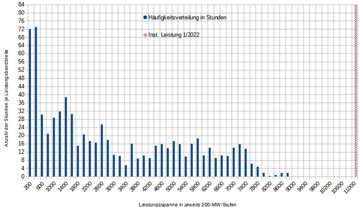
Häufigkeitsverteilung der Leistungsbandbreiten nach Daten von Amprion
