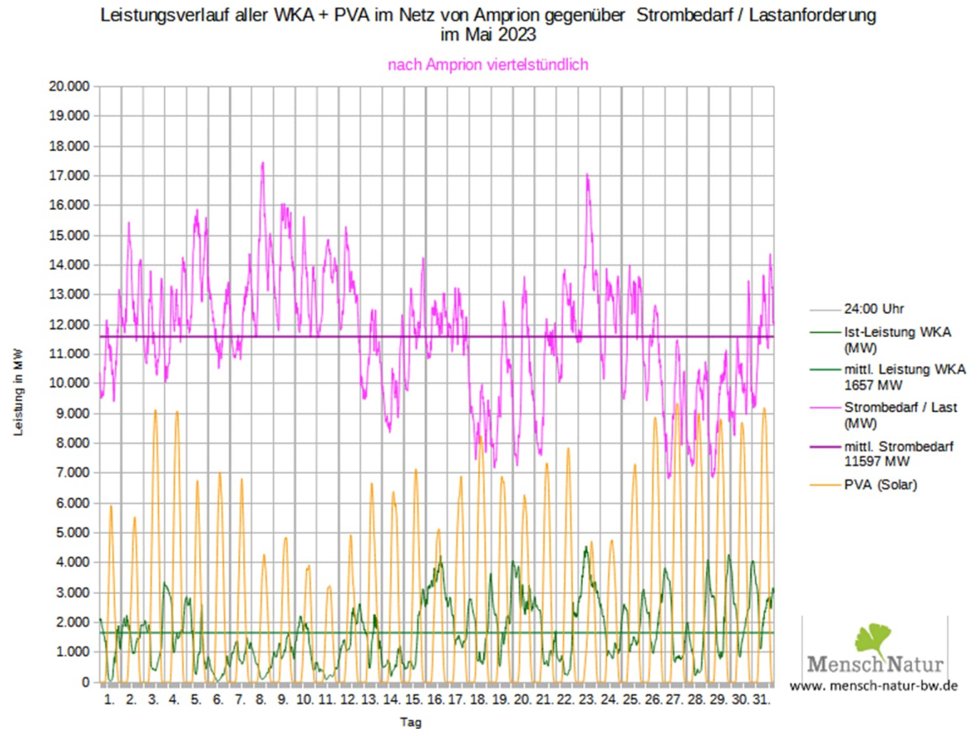
Leistungsverlauf Windleistung gegen Strombedarf (Last) Amprion
