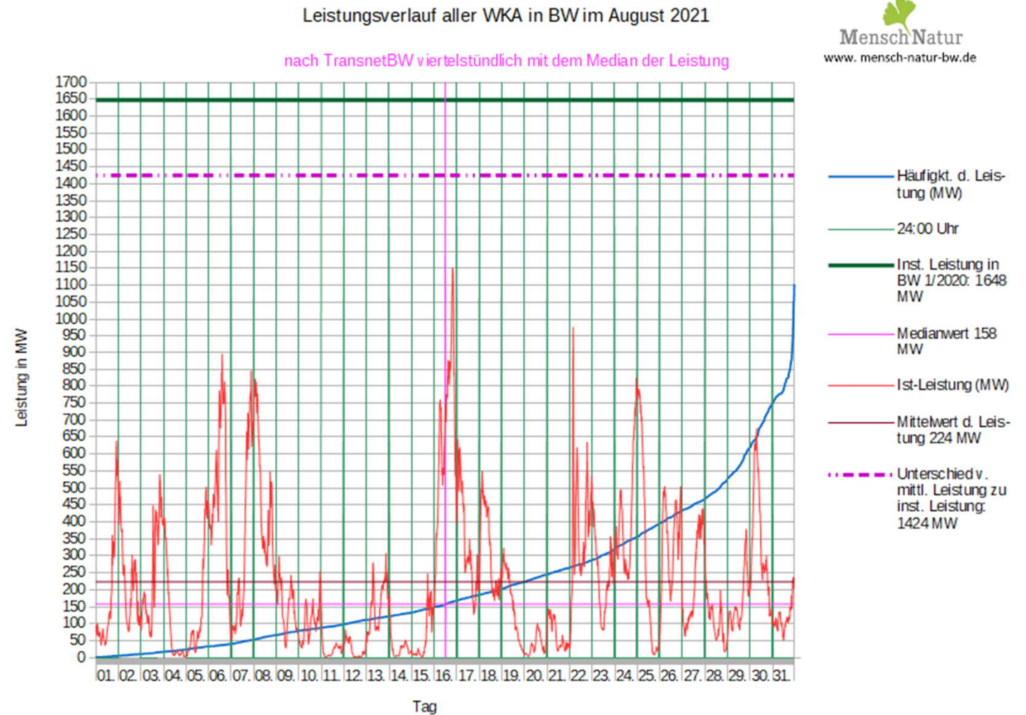
Analyse der Leistungsverteilung von Windenergie zur installierten Leistung TransnetBW
