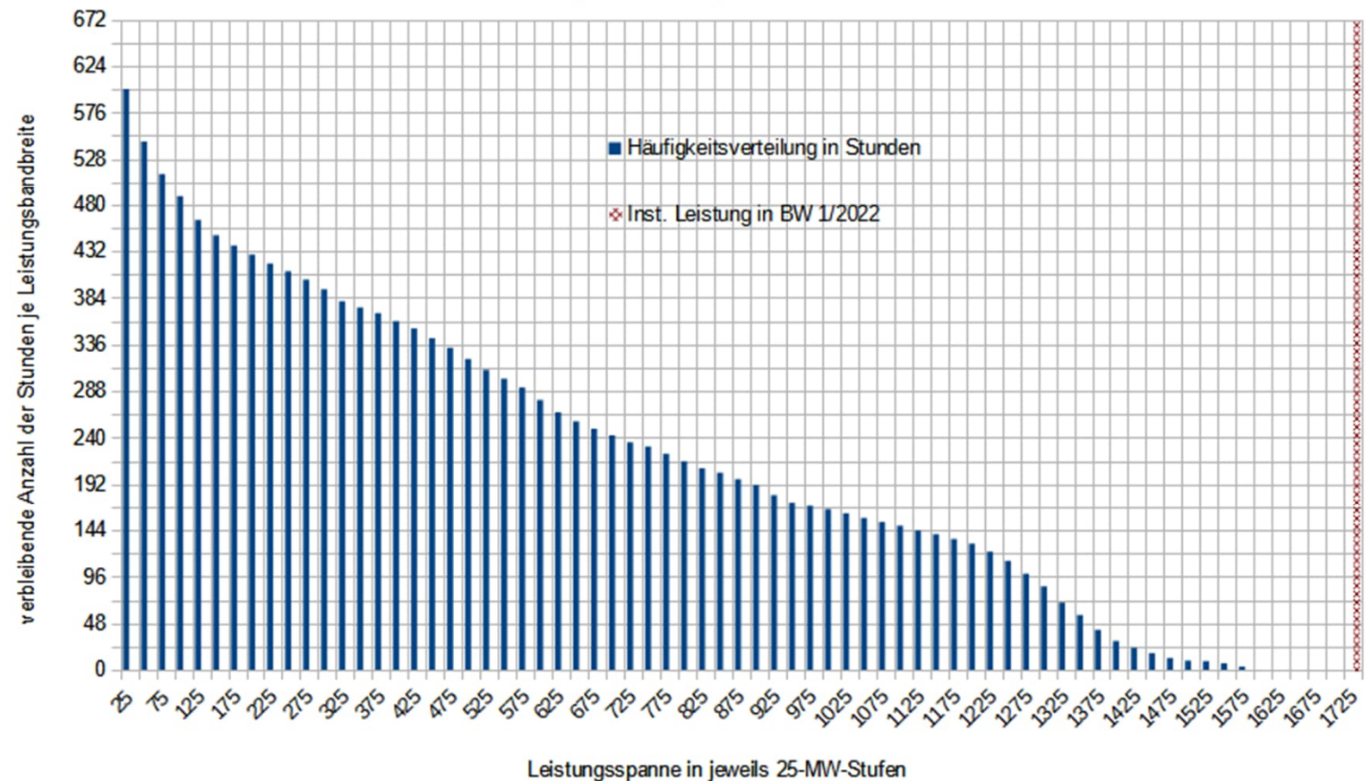
Häufigkeitsverteilung über die monatliche Gesamtstunden mit verfügbaren Leistungsstufen in Stunden TransnetBW
