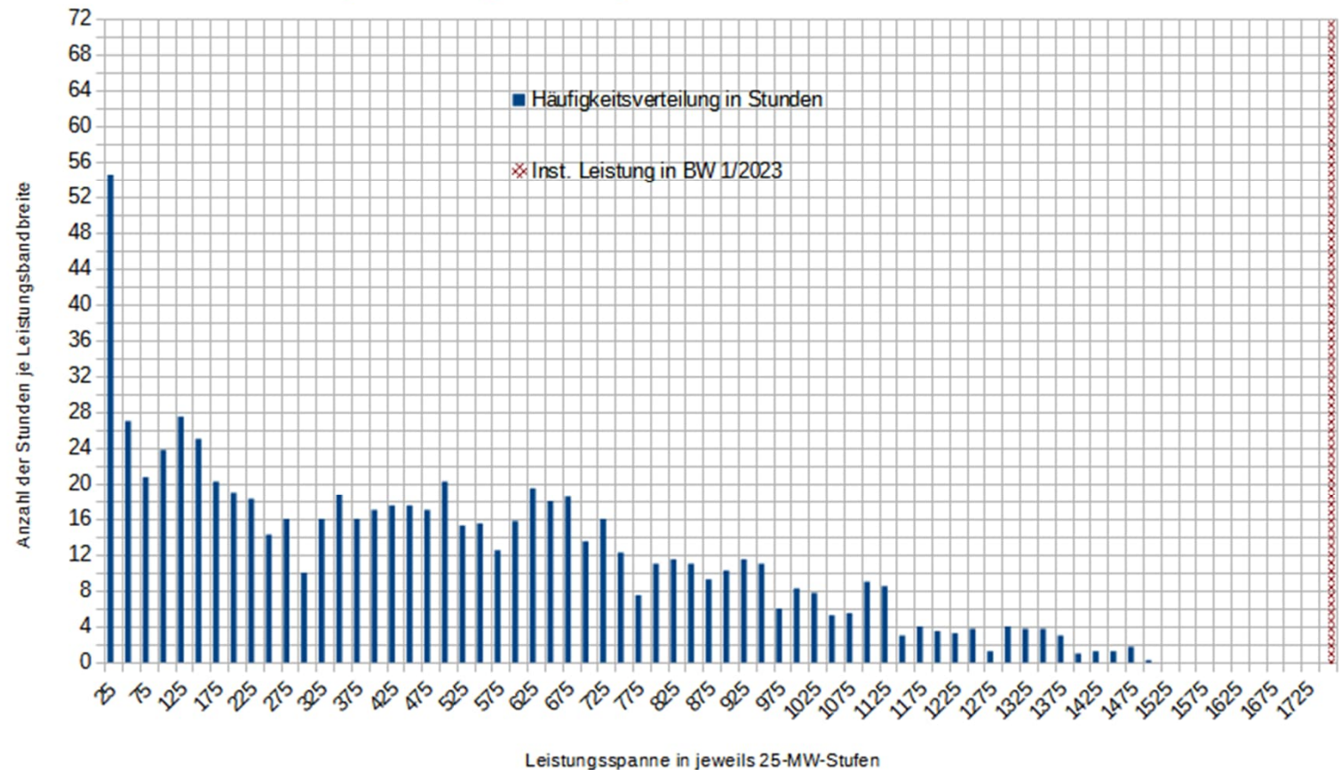
Häufigkeitsverteilung der Leistungsbandbreiten nach Daten von TransnetBW
