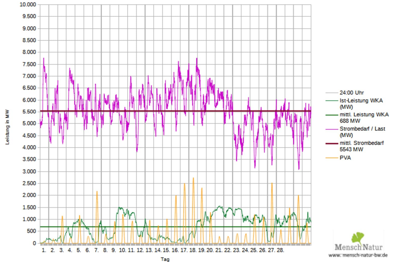
Leistungsverlauf Windleistung gegen Strombedarf (Last) TransnetBW
