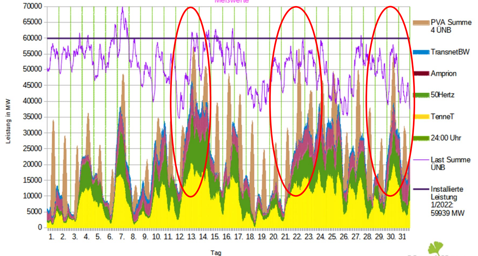
Strombedarf ("Last") und erbrachte Leistung aller PVA und WKA in D an Land + auf See im März 2023
