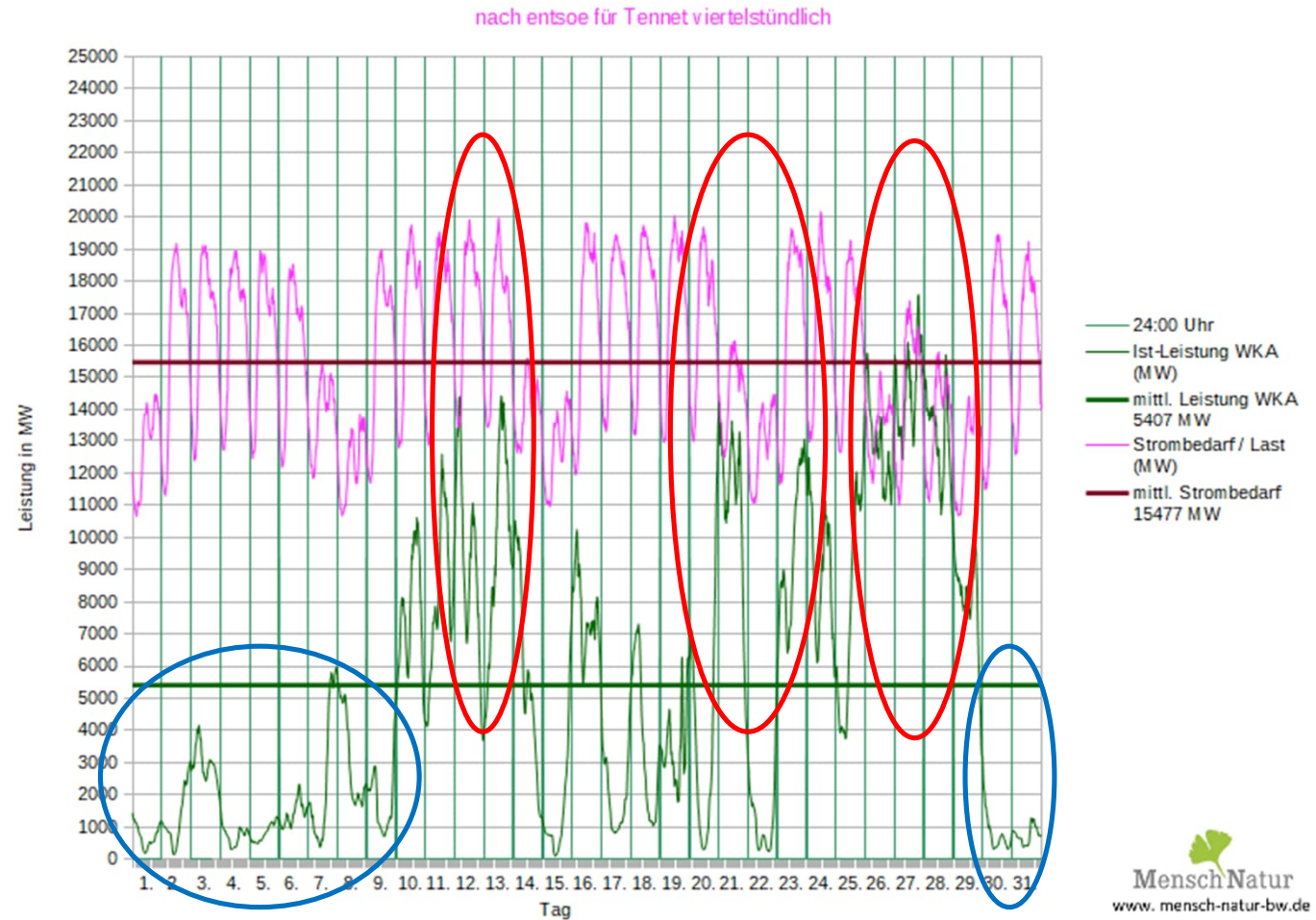
Leistungsverlauf Windleistung gegen Strombedarf (Last) Tennet
