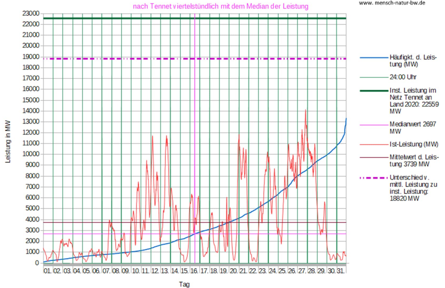
Leistungsverlauf aller WKA an Land im Netz Tennet im Mai 2022
