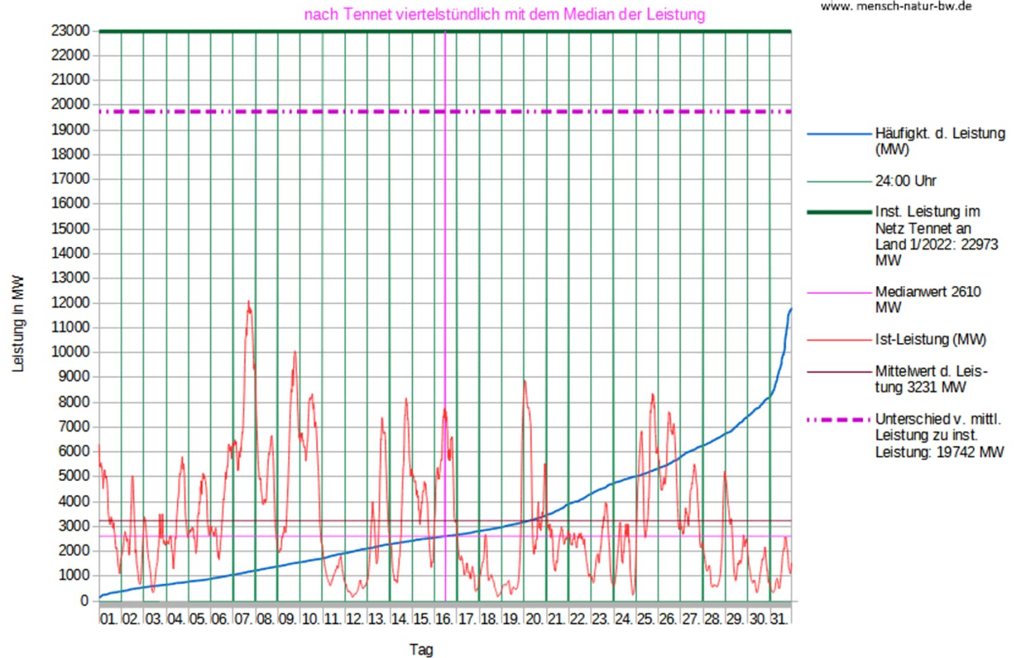
Leistungsverlauf aller WKA an Land im Netz Tennet im Juli 2022
