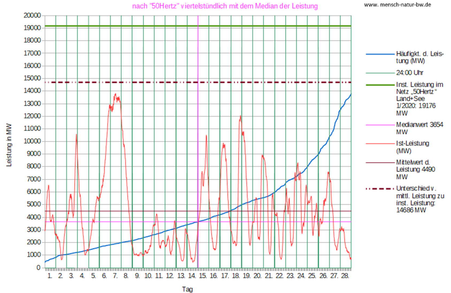
Leistungsverlauf aller WKA an Land + See im Netz "50Hertz" im Februar 2021
