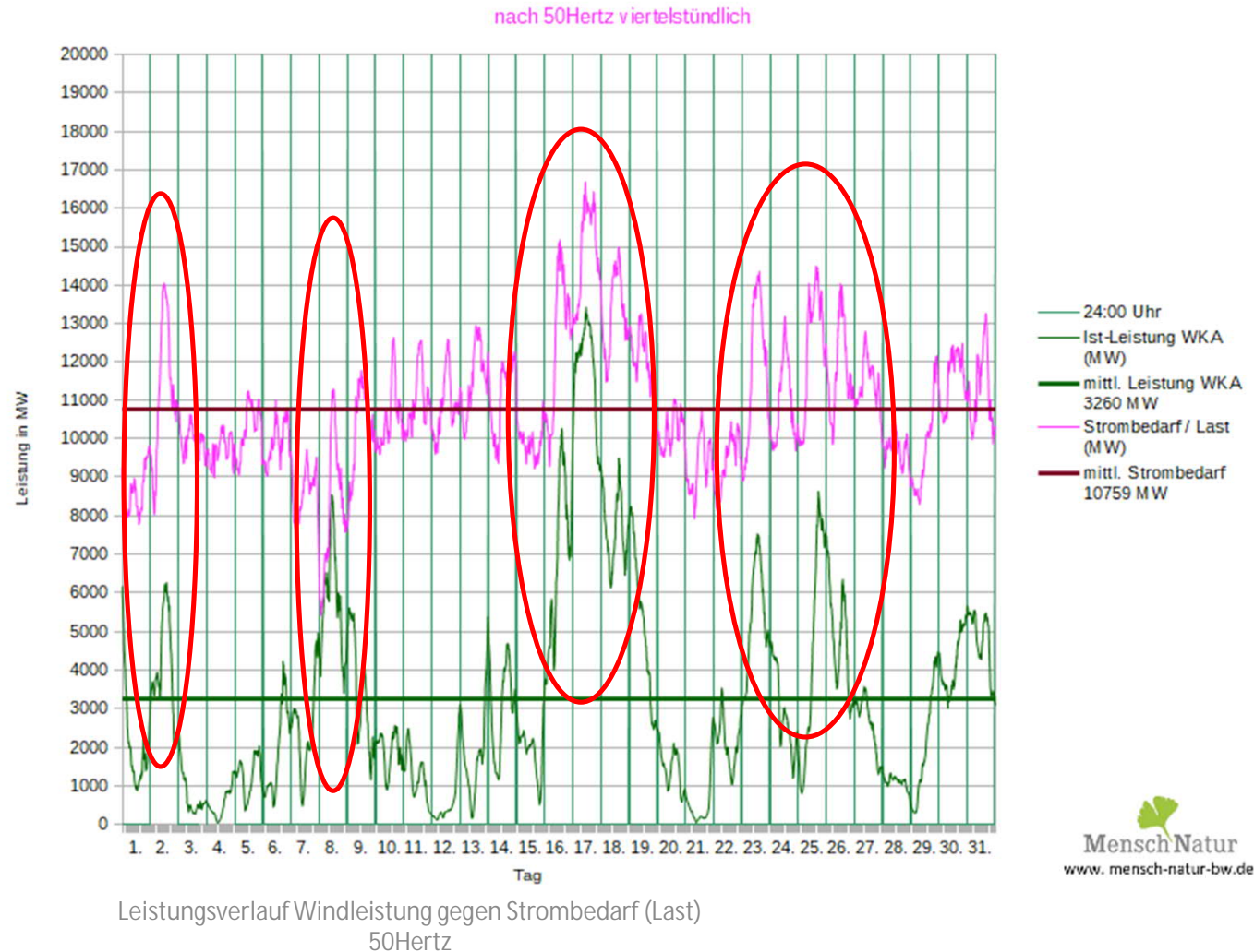
Leistungsverlauf aller WKA in 50Hertz gegenüber Strombedarf / Lastanforderung im August 2021
