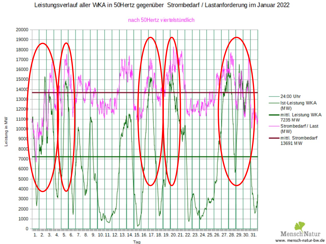
Leistungsverlauf Windleistung gegen Strombedarf (Last) 50Hertz
