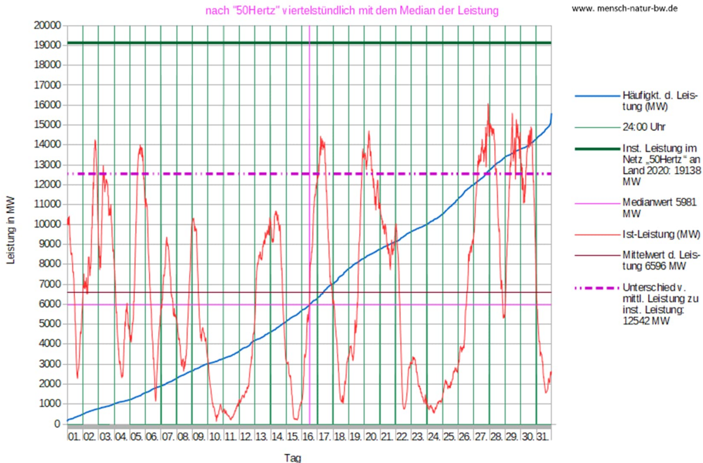
Analyse der Leistungsverteilung von Windenergie an Land zur installierten Leistung 50Hertz
