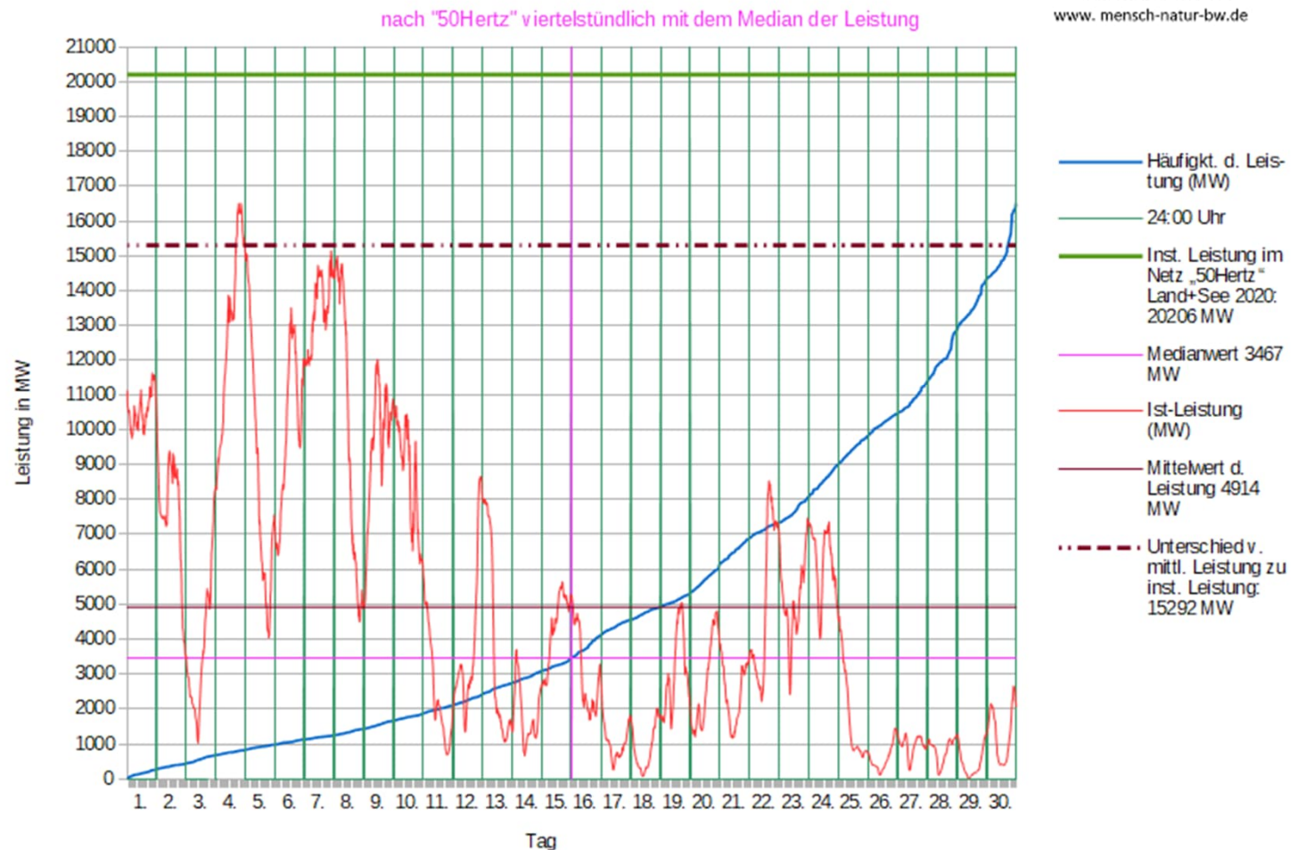
Leistungsverlauf aller WKA an Land + See im Netz "50Hertz" im April 2022
