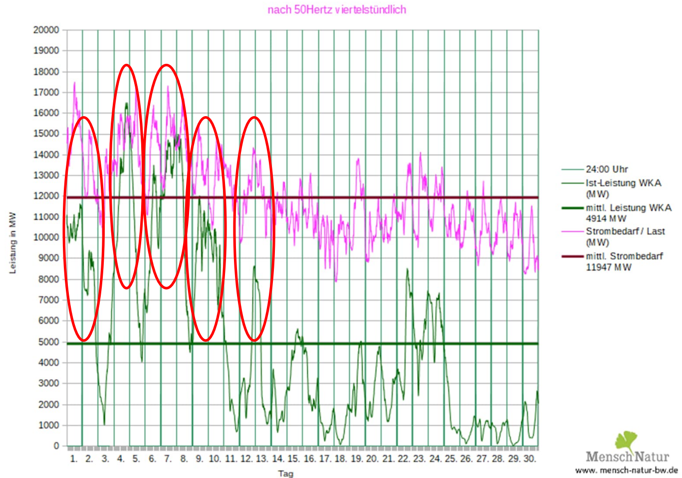
Leistungsverlauf aller WKA in 50Hertz gegenüber Strombedarf / Lastanforderung im April 2022
