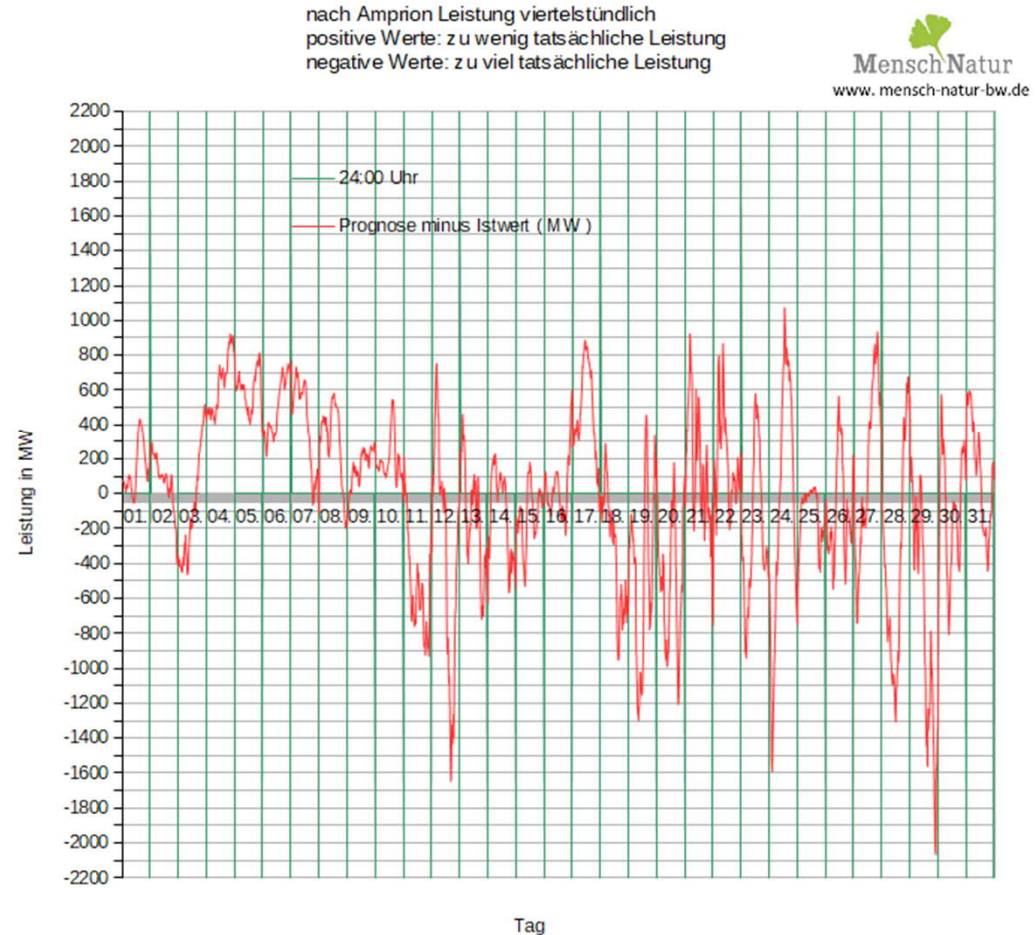
Differenz zw. Prognose der Leistung zu tatsächlicher Leistung in MW im Januar 2021
