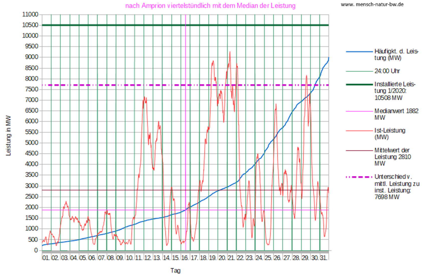
Leistungsverlauf aller WKA im Netz von Amprion im Januar 2021
