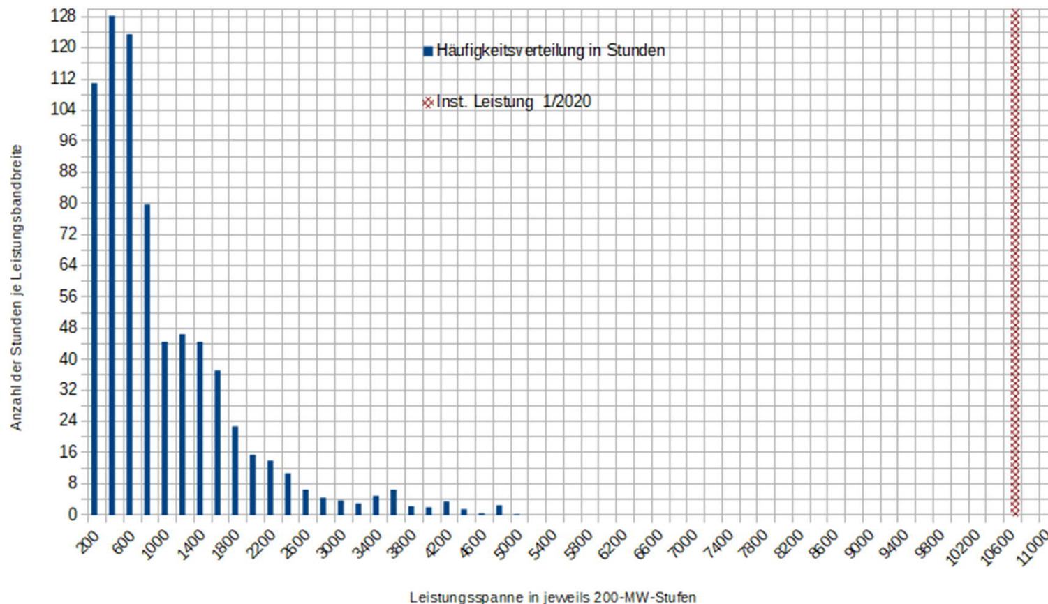
Häufigkeitsverteilung der Leistung Amprion
