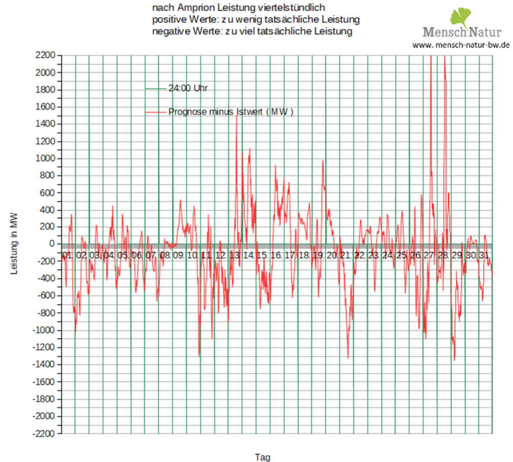
Differenz zw. Prognose der Leistung zu tatsächlicher Leistung in MW im März 2021
