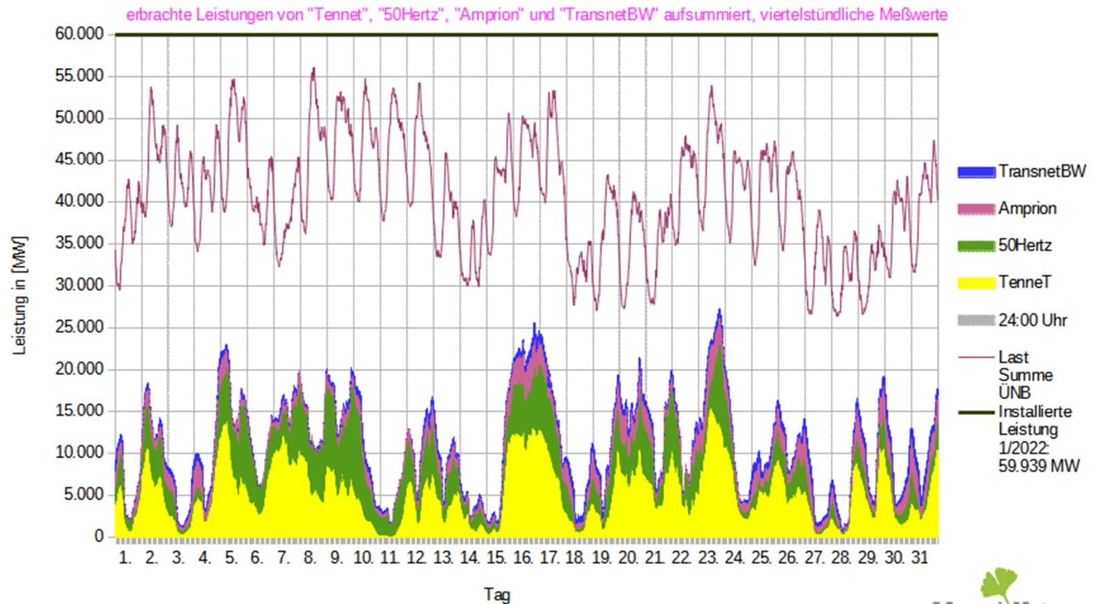
Strombedarf („Last“) und tatsächlich erbrachte Leistung aller WKA in D an Land + auf See im Mai 2023
