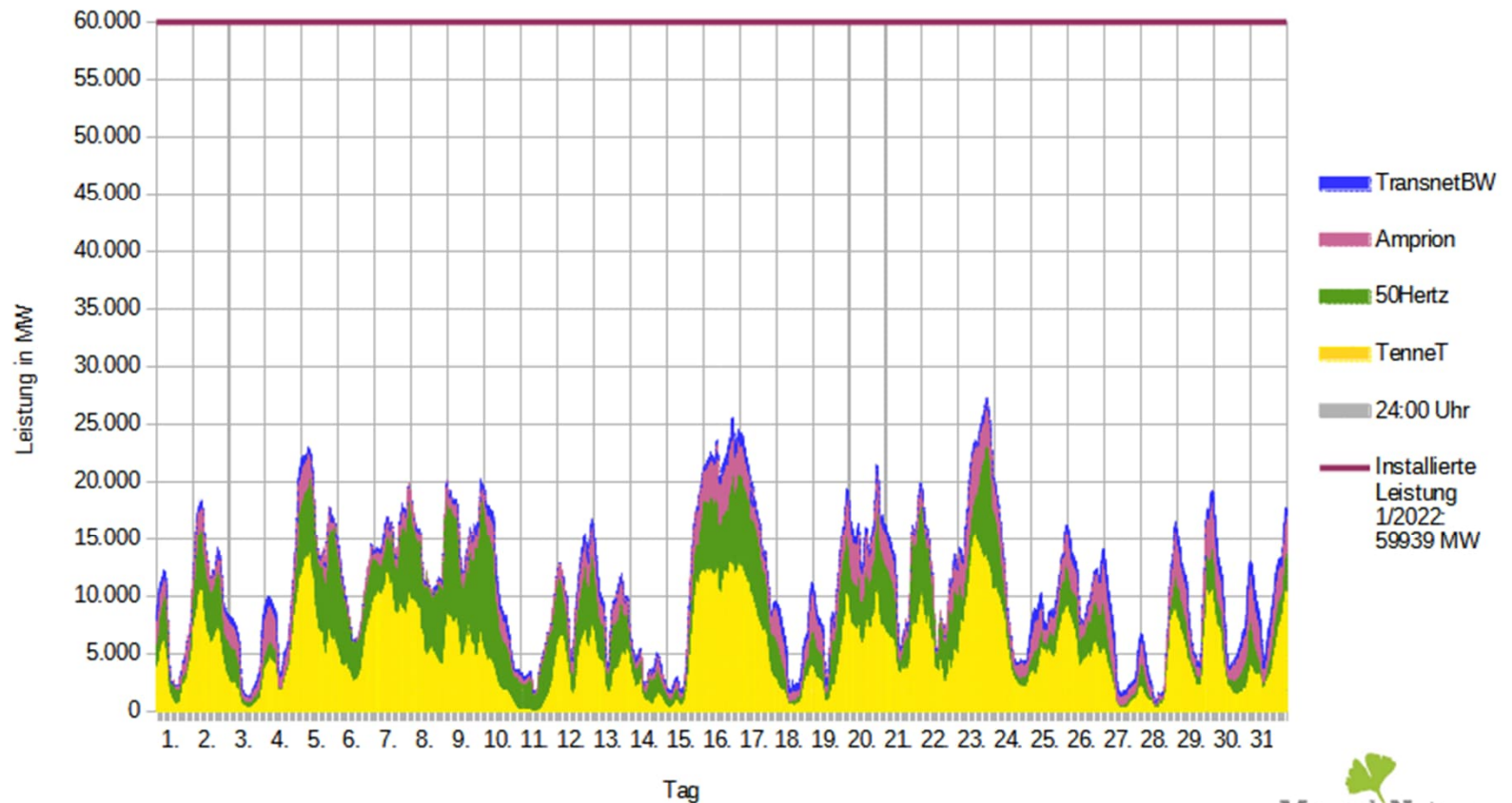
Tatsächlich erbrachte Leistung aller WKA in D an Land + auf See im Mai 2023 erbrachte Leistungen von „TenneT“, „50Hertz“, „Amprion“ und „TransnetBW“ aufsummiert, viertelstündliche Meßwerte
