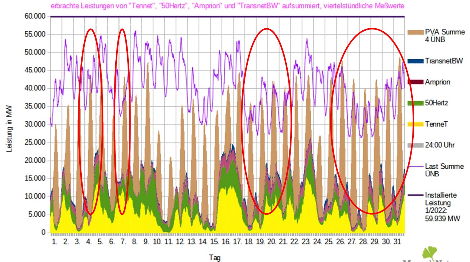
Strombedarf („Last“) und erbrachte Leistung aller PVA und WKA in D an Land + auf See im Mai 2023
